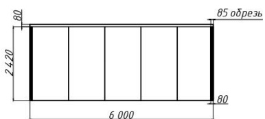
Фронтальная сторона
