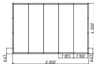
Пол
